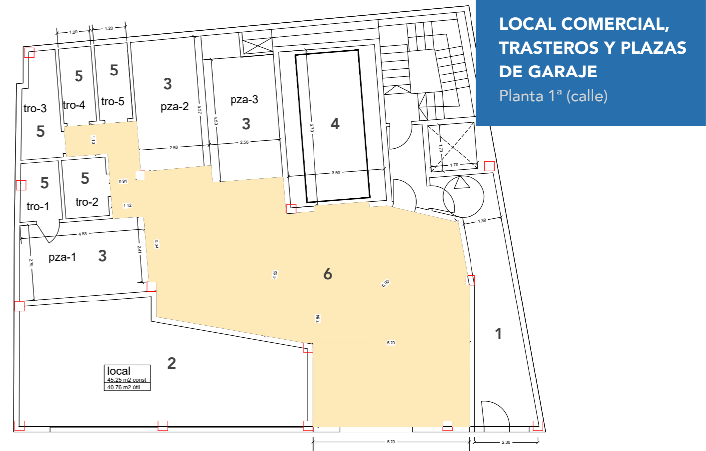
1. Vestíbulo 2. Local Comercial 3. Plazas de garaje 4. Ascensor de vehículos 5. Trasteros 6. Acceso de vehículos Superficie construida Local Comercial: 45,25 m 2
